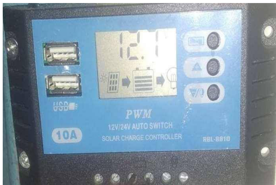
Gambar 4. 1 Monitor Sistem Panel Surya pada Modul SCC
