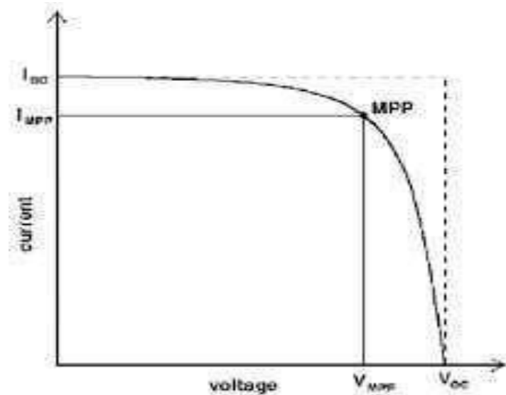
Gambar 2.7 Kurva Karakteristik V-I pada Sel Surya Sumber : Rafika A, 2017
