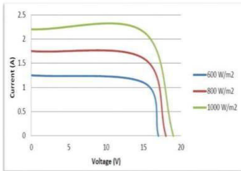
Gambar 2.12 Grafik arus dan tegangan terhadap insolation
