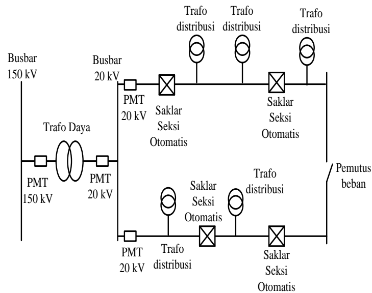
Gambar 2.3 Pola Jaringan Loop
