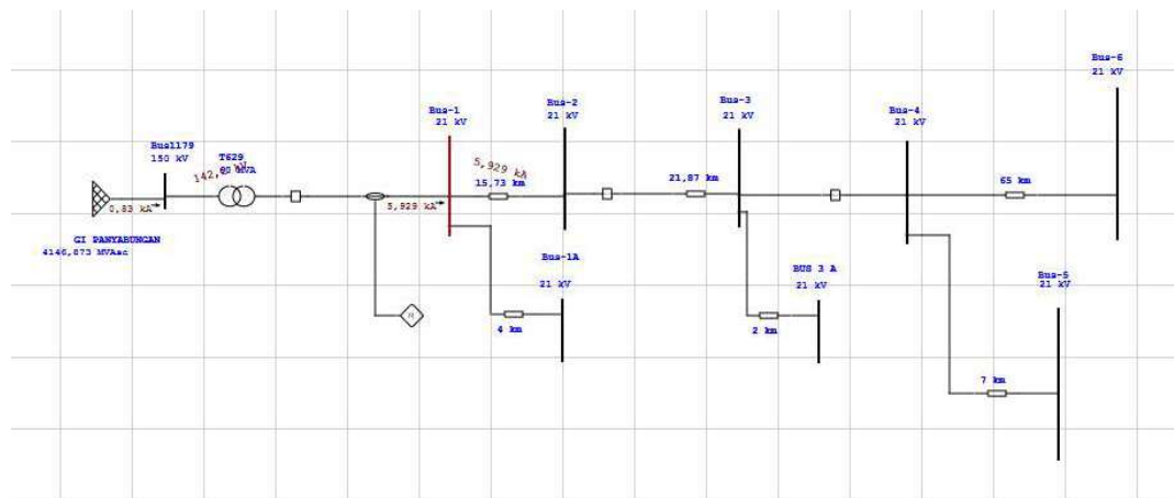
Gambar 4.33 Simulasi Hubung Singkat 3 Fasa Pada Lokasi 1
