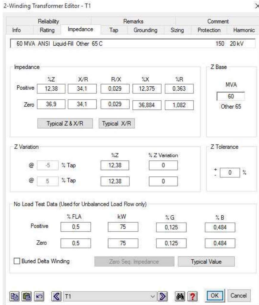
Gambar 4.17 Setting Impedansi Transformator Step Down 60 MVA Sumber: Penulis, 2020
