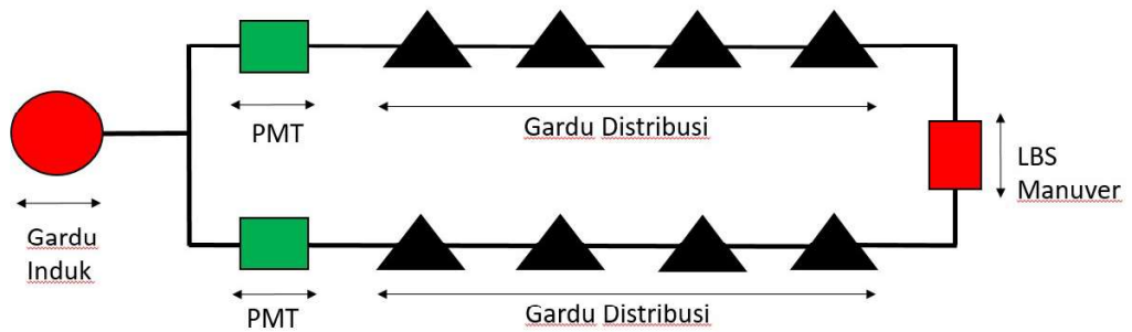
Gambar 2.6 Konfigurasi Jaringan Tertutup/loop
