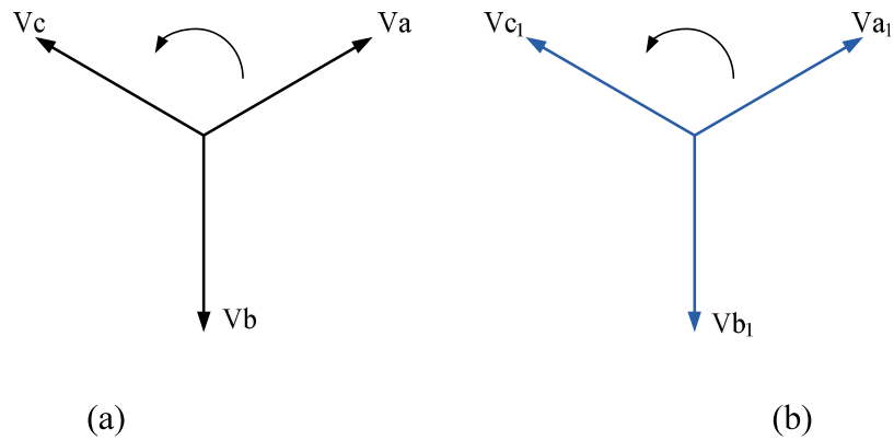
Gambar 2.13 (a) Urutan Fasor Asli dan (b) Komponen Urutan Positif Sumber : PT. PLN (Persero) Pusdiklat “Konsep Dasar Jaringan Distribusi” Materi Pembedangan Bidang Operasi Distribusi Edisi 1, 2012
