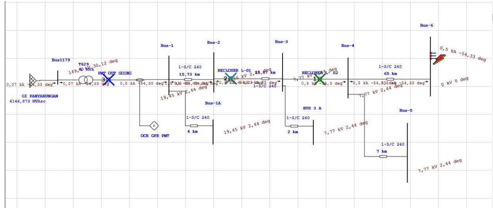
Gambar 4.46 Simulasi Koordinasi Peralatan Proteksi Dalam Mengamankan Gangguan 3 Fasa Pada Lokasi 3 Sumber: Penulis, 2020
