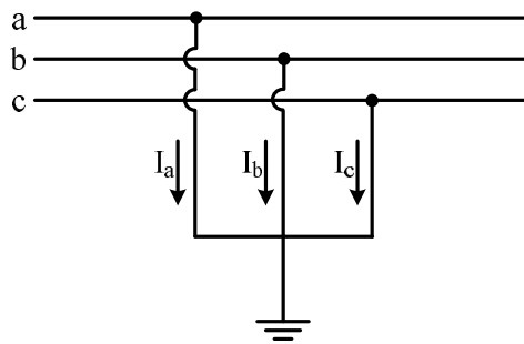
Gambar 2.24 Diagram Rangkaian Gangguan Hubung Singkat Tiga Fasa atau Tiga Fasa ke Tanah
