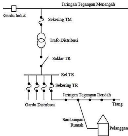
Gambar 2.3 Sistem Distribusi Sekunder
