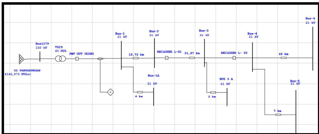
Gambar 4.11 Daerah 1 Penyulang YB-02
