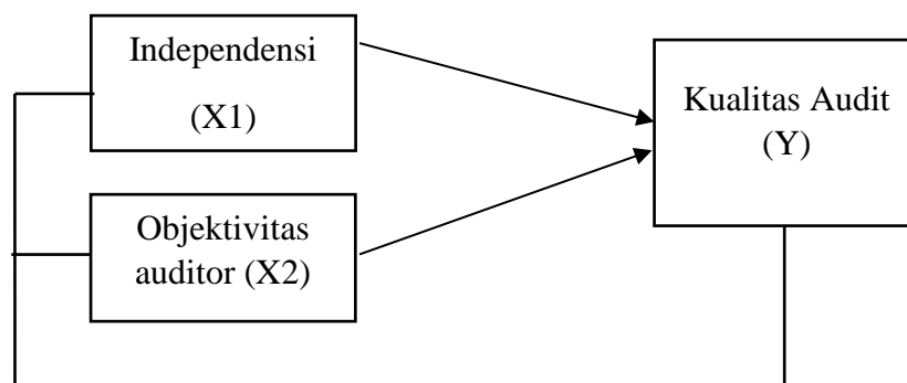
Gambar 2.1 Kerangka Konseptual
