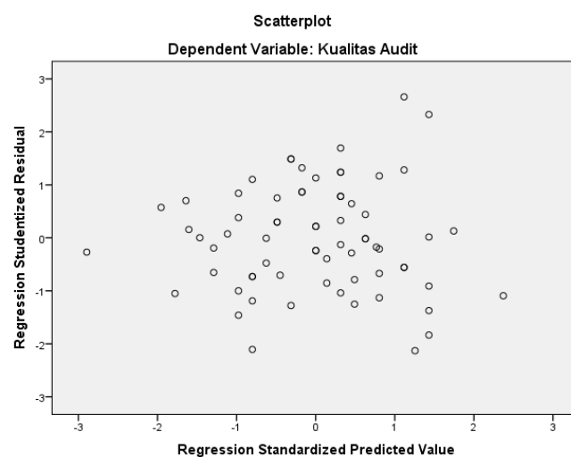
Gambar 4.4 Uji Heteroskedastisitas
