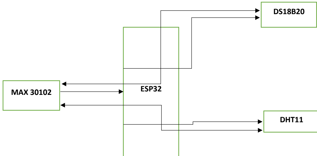
Gambar 3.2 Diagram blok perangkat keras
