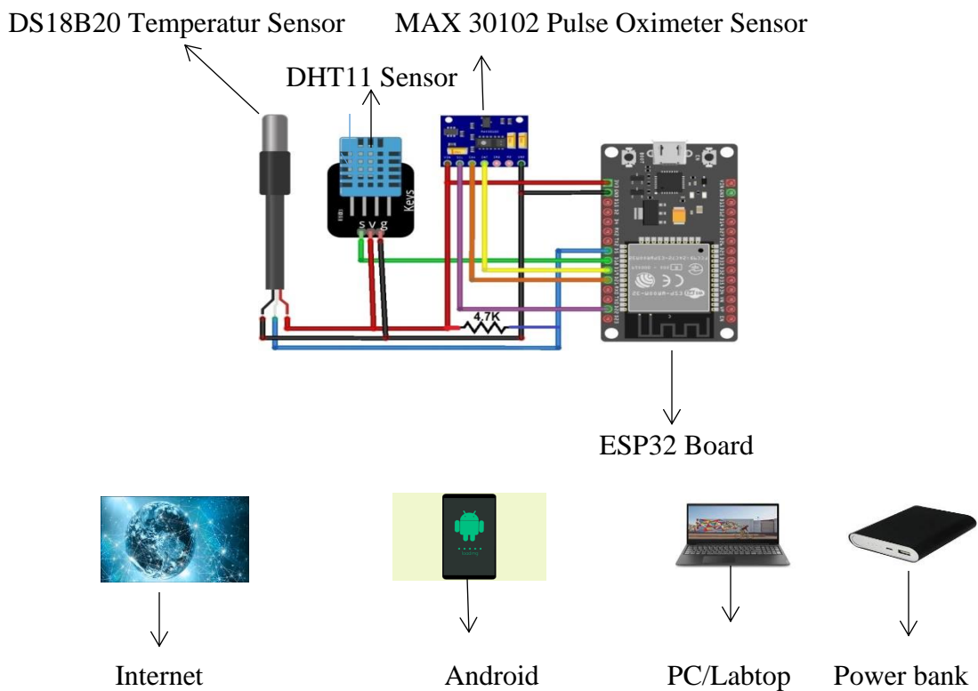
Gambar 3.1 Perancangan sistem pemantauan kesehatan
