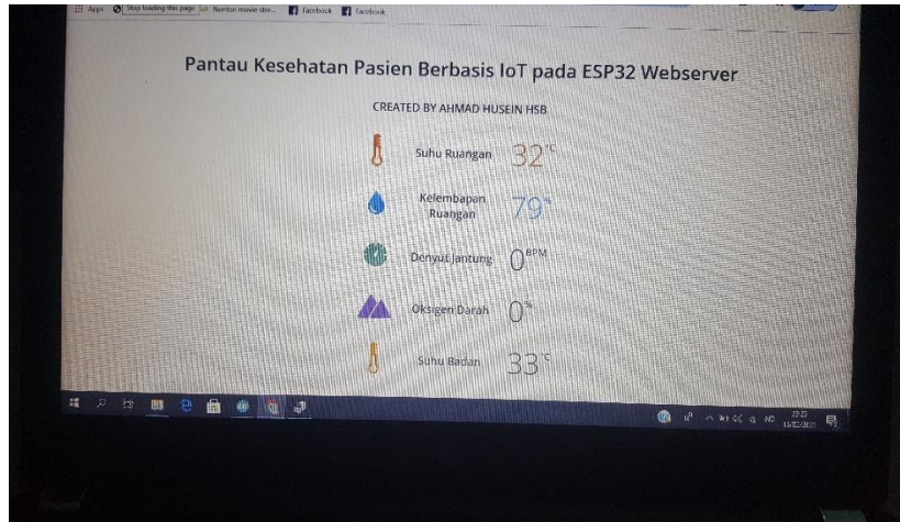
Gambar 4.6 Hasil pengujian DS18B20/sudah di ganti ke DHT11 ialah 33 derajat celcius.
