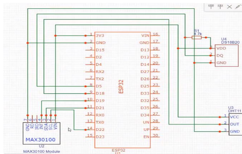
Gambar 3.2 Rancangan perangkat keras keseluruhan
