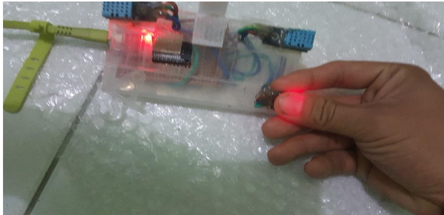
Gambar 4.2 Pengujian MAX 30102
