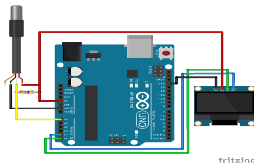
Gambar 2.5 DS18b20 Sumber : symask.blogspot
