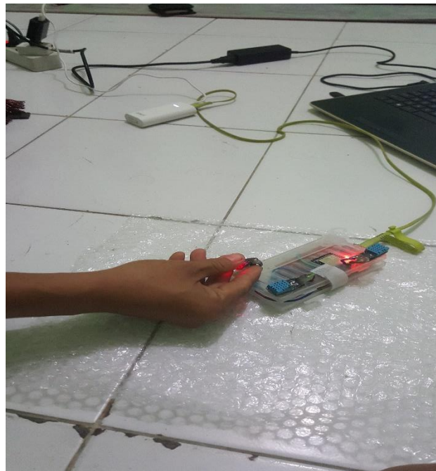
Gambar 4.4 pengujian sensor DHT11
