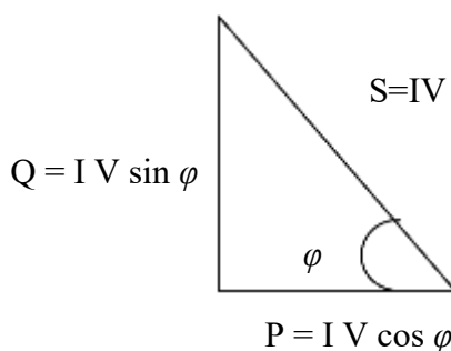
Gambar 2.1.1 Segitiga Daya
