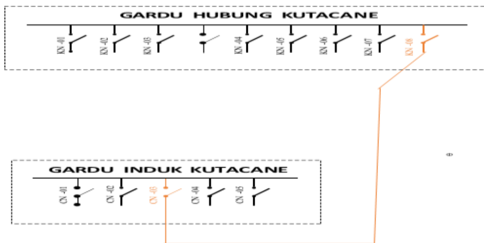
Gambar 3.6.1 Diagram Alir Gardu Induk Ke Gardu Hubung
